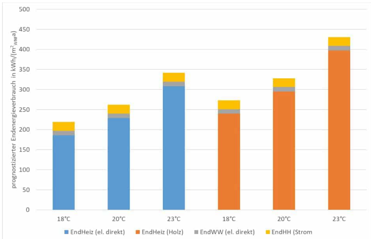
Abbildung 60: spezifischer Endenergieverbrauch des größeren Gebäudes vor Sanierung gemäß Verbrauchsprognoseberechnungen PHPP unter Annahme unterschiedlicher Mittelwerte der Raumlufthtemperatur in der Heizperiode für eine direkt-elektrische Beheizung aller Wohnungen und eine Beheizung aller Wohnungen über Holzöfen
