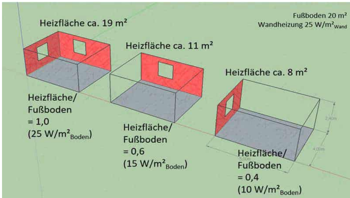
Abbildung 88: Wärmeabgabefläche der Wandheizung im Verhältnis zur Fußbodenfläche verschiedener Räume ( 4 \times 5 \text{ m} = 20 \text{ m}^2 ; Höhe 2.4 \text{ m} , spezifische Wärmeabgabeleistung der Wandheizung 25 \text{ W/m}^2_{\text{Wand}} )
