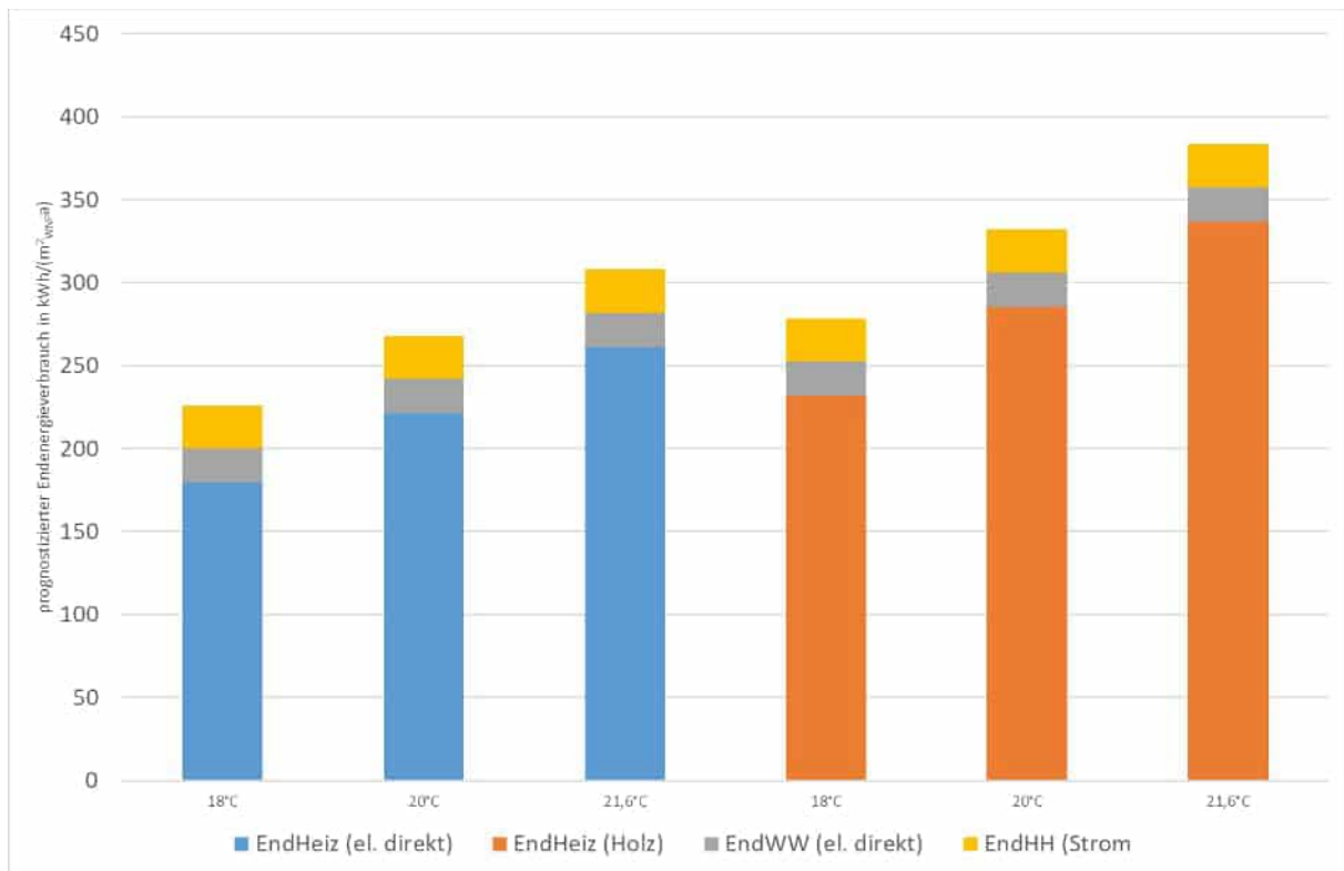
Abbildung 61: spezifischer Endenergieverbrauch des kleineren Gebäudes vor Sanierung gemäß Verbrauchsprognoseberechnungen PHPP unter Annahme unterschiedlicher Mittelwerte der Raumlufttemperatur in der Heizperiode für eine direkt-elektrische Beheizung aller Wohnungen und eine Beheizung aller Wohnungen über Holzöfen
