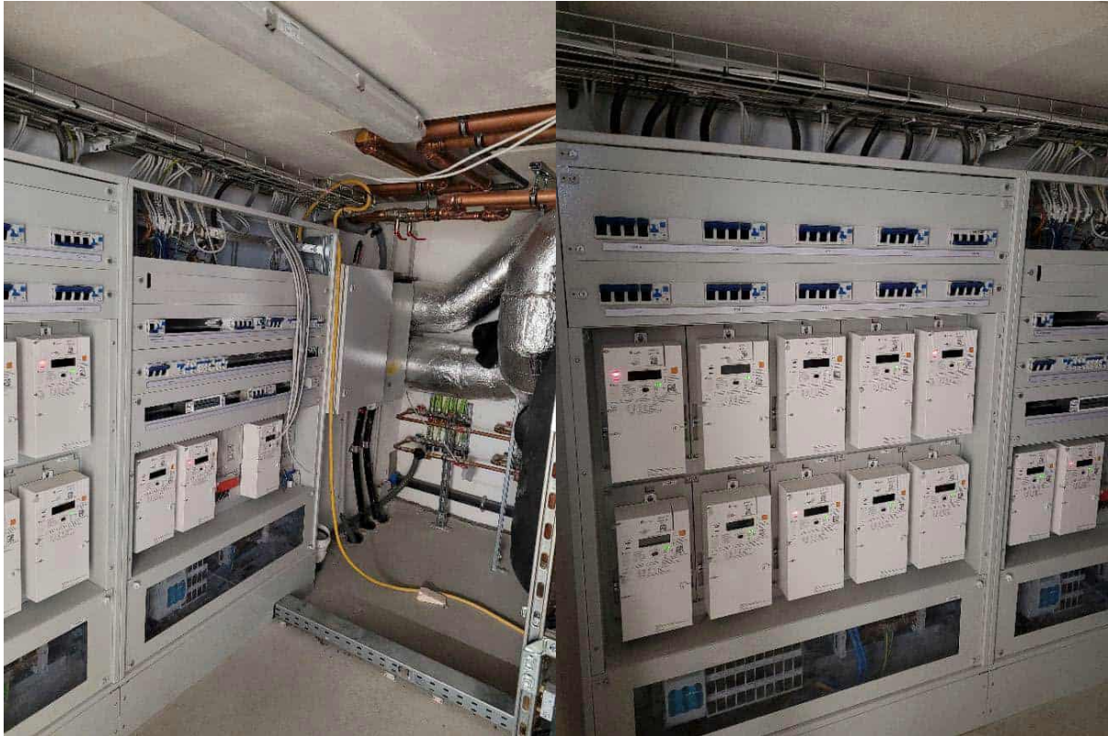
Abbildung 141: Elektrozähler im Kellergeschoß; Fotos: Energieinstitut Vorarlberg
