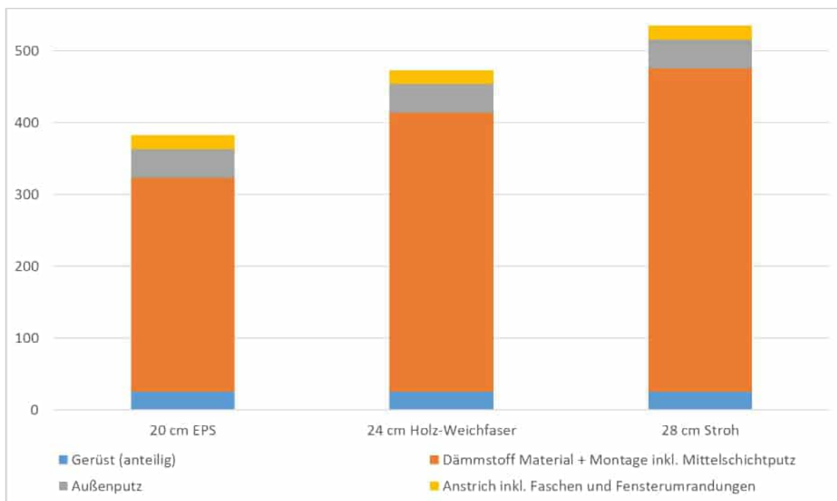
Abbildung 216: spezifische Kosten verschiedener energetisch gleichwertiger Varianten der nachträglichen Außenwanddämmung mit Wärmedämm-Verbundsystem (netto, in EUR/m 2 Bauteilfläche)
