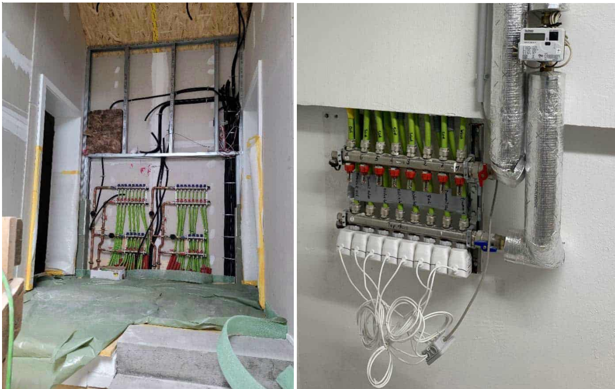
Abbildung 128: Außenwandheizungs-Heizkreisverteiler im Treppenhaus DG (links), Foto: Rhomberg Bau GmbH und im Kellergeschoß, Foto: Energieinstitut Vorarlberg
