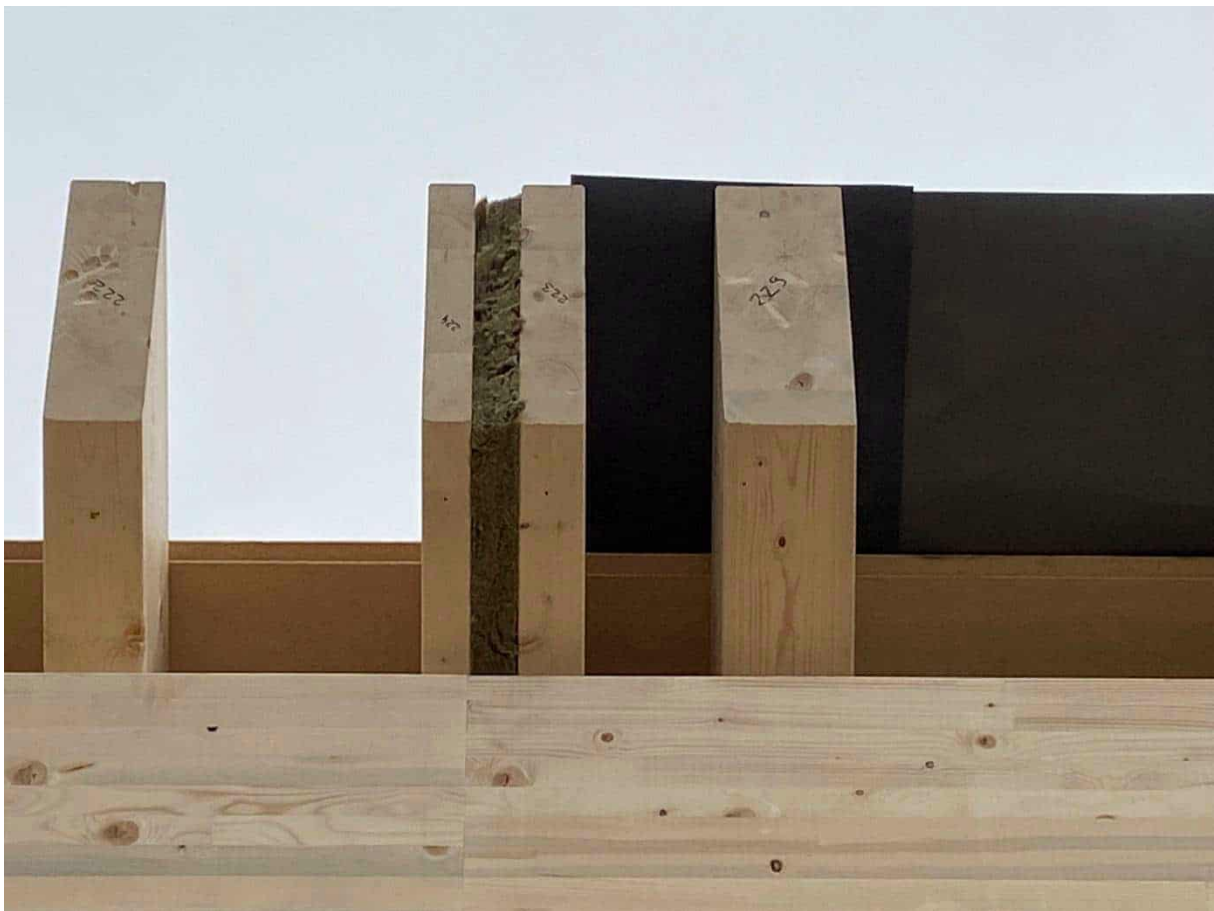
Abbildung 179: kleines Gebäude: Stoß der vorgefertigten Dachelemente, Foto: Rhomberg Bau GmbH
