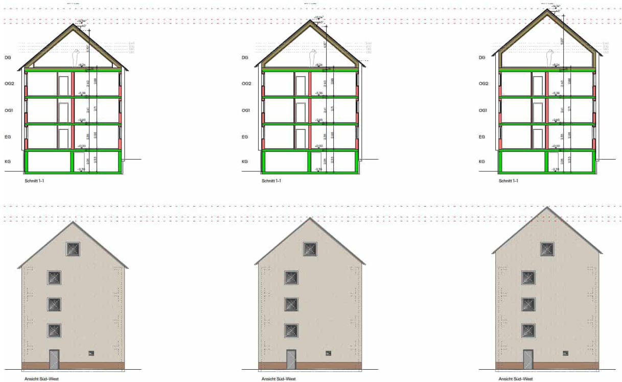
Abbildung 72: Schnitte und Ansichten Süd-West der Entwurfsvarianten für das Dachgeschoß des größeren Gebäudes - ohne Aufschiebling, ohne Kniestock sowie mit zwei Kniestockhöhen; Johannes Kaufmann und Partner GmbH
