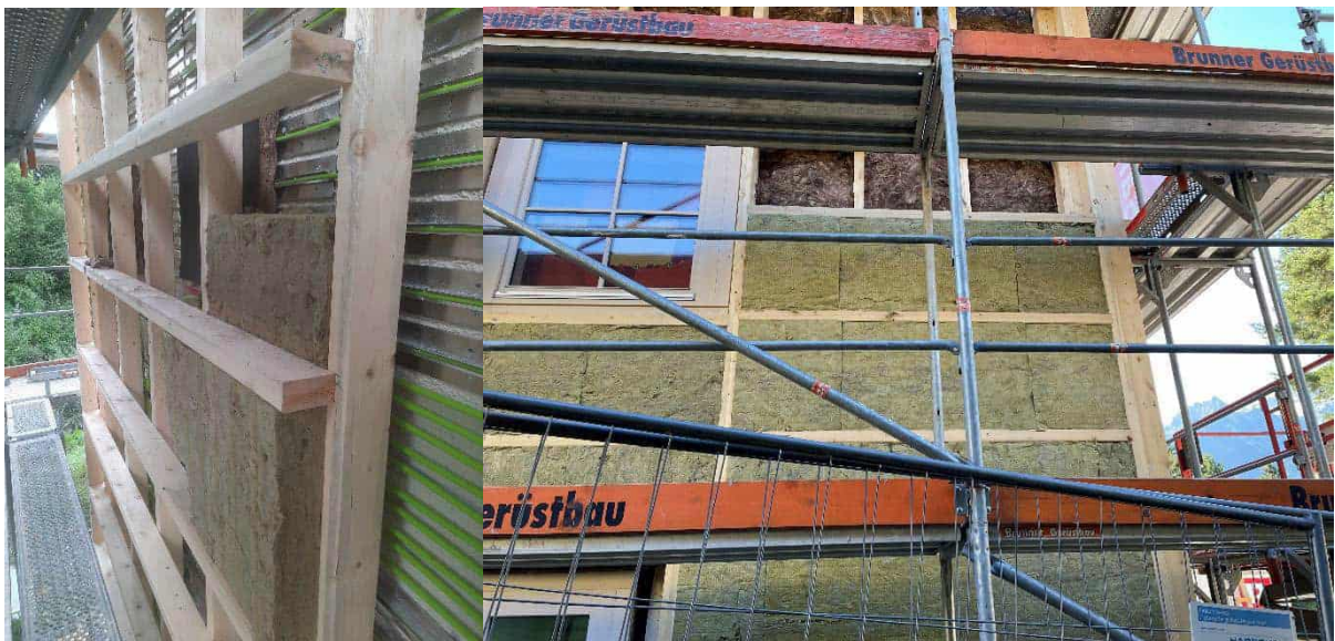
Abbildung 112: großes Gebäude: erste und zweite Lage Mineralwolldämmung; Fotos: Energieinstitut Vorarlberg
