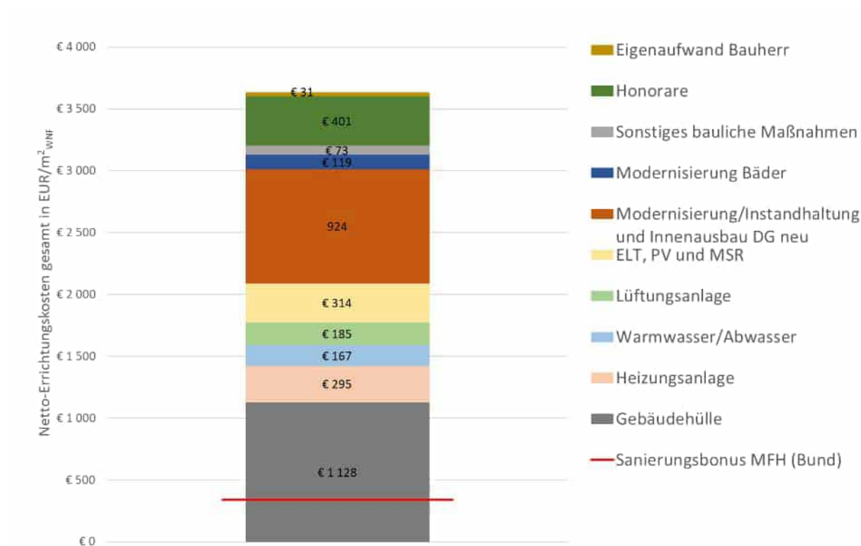
Abbildung 206: abgerechnete, wohnflächenspezifische Netto-Errichtungskosten des großen Gebäudes
