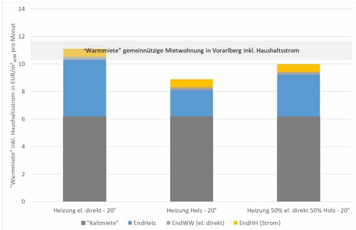
Abbildung 3: monatliche Warmmiete inkl. Haushaltsstrom für Mieter*innen mit befristetem Mietvertrag, abhängig von der Art der Beheizung und unter Annahme einer mittleren Heizperioden-Raumlufttemperatur von 20°C (größeres Gebäude); Vergleichskosten für gemeinnützige Neubauten in Vorarlberg (grauer Balken)
