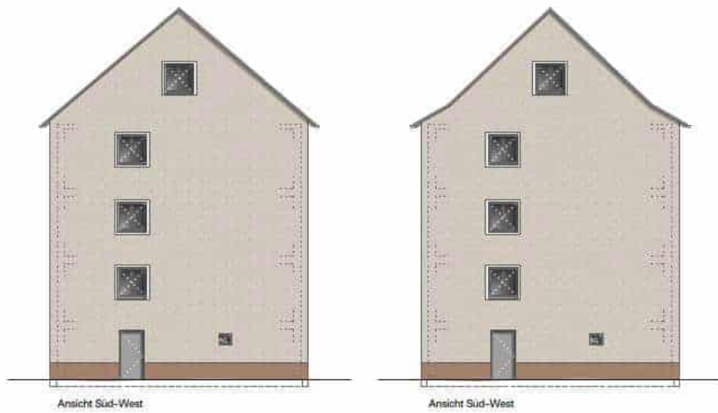
Abbildung 70: Entwurfsvarianten Dachgeschoß größeres Gebäude ohne Kniestock, mit und ohne Aufschiebling; Johannes Kaufmann und Partner GmbH
