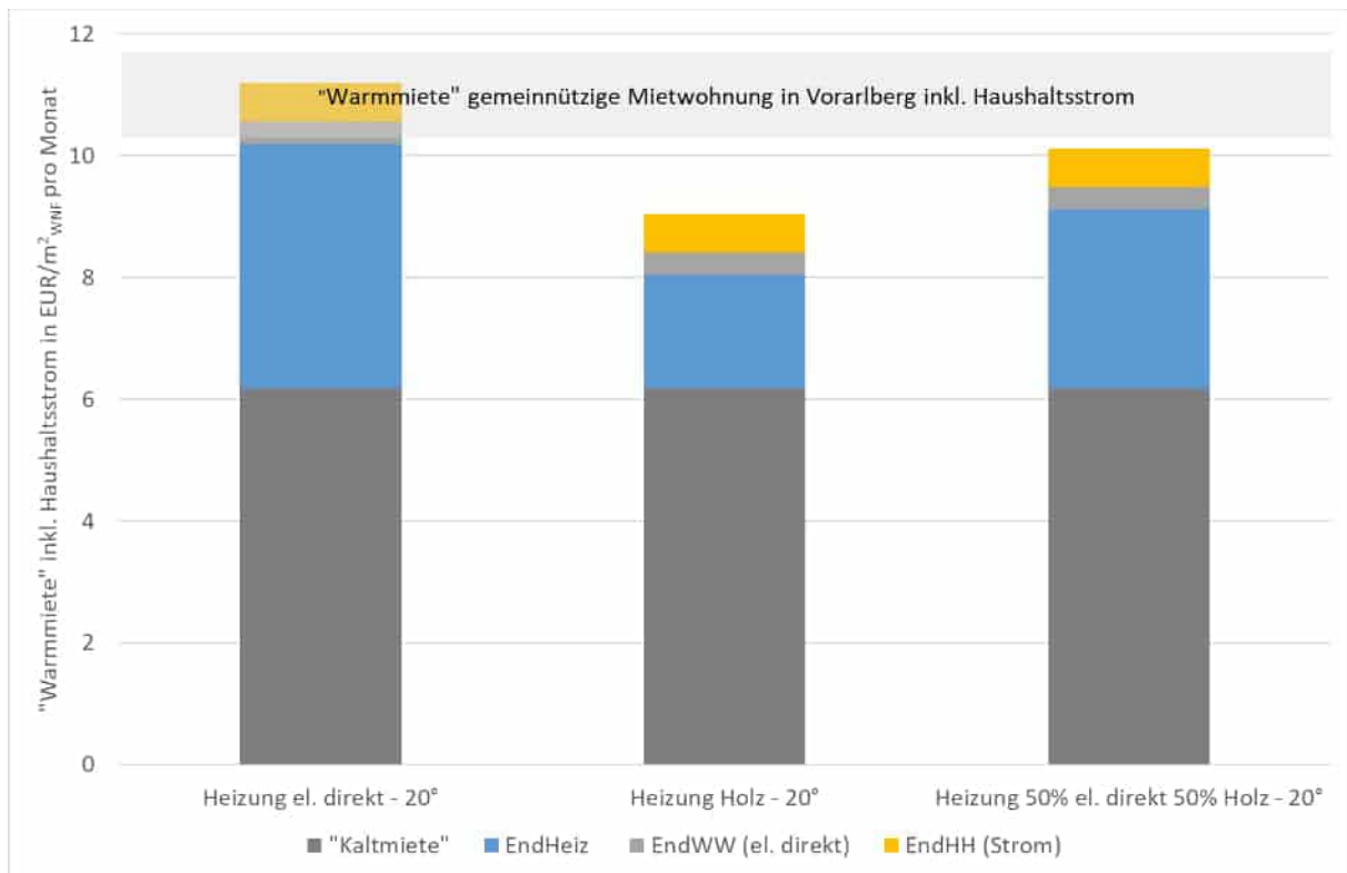
Abbildung 68: monatliche Warmmiete inkl. Haushaltsstrom für Mieter*innen mit befristetem Mietvertrag in Abhängigkeit von der Art der Beheizung und unter Annahme einer mittleren Heizperioden-Raumlufthtemperatur von 20°C – kleines Gebäude; Vergleichskosten für gemeinnützige Neubauten in Vorarlberg
