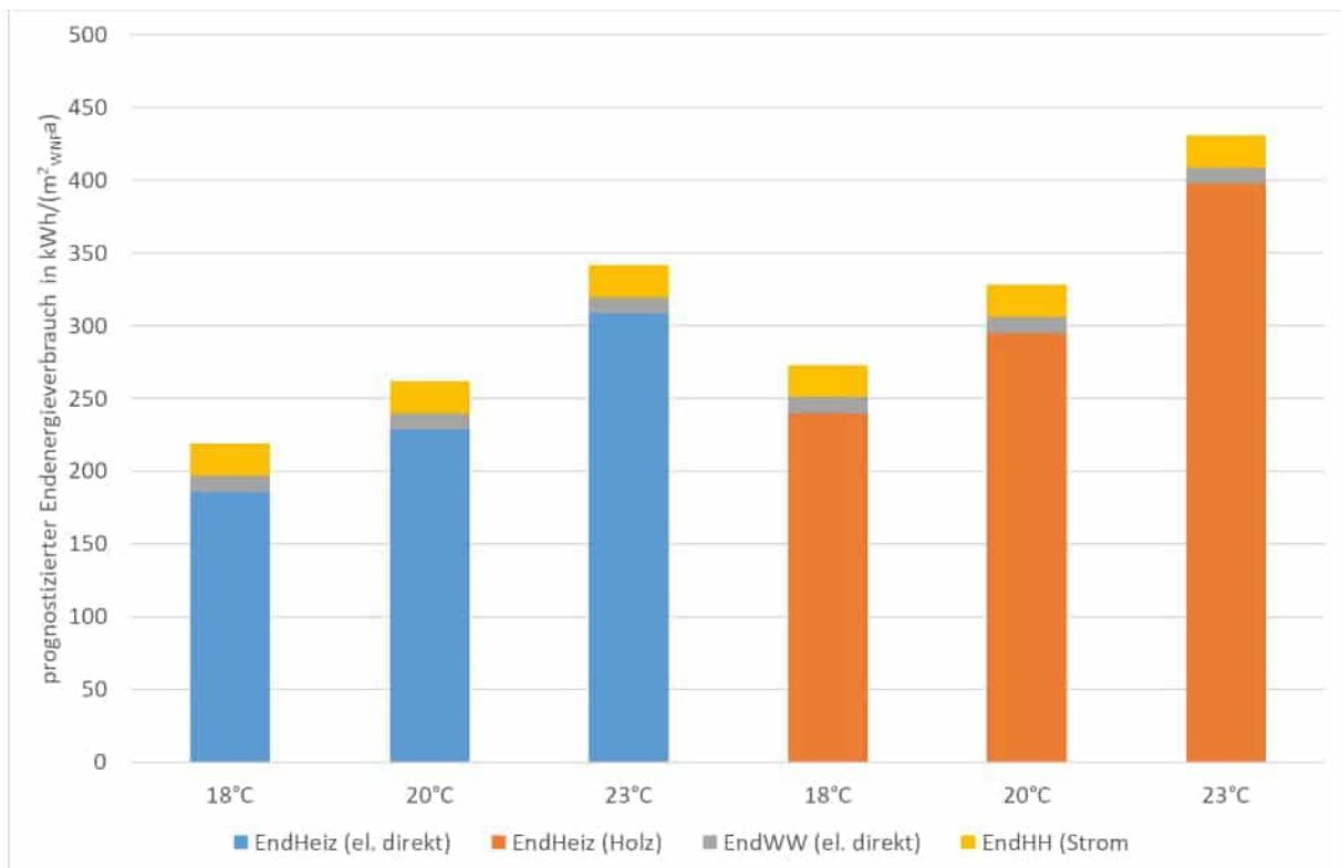
Abbildung 2: Spezifischer Endenergieverbrauch des großen Gebäudes vor der Sanierung gemäß Verbrauchsprognoseberechnungen mit PHPP. Dargestellt sind die Werte für eine direkt-elektrische
