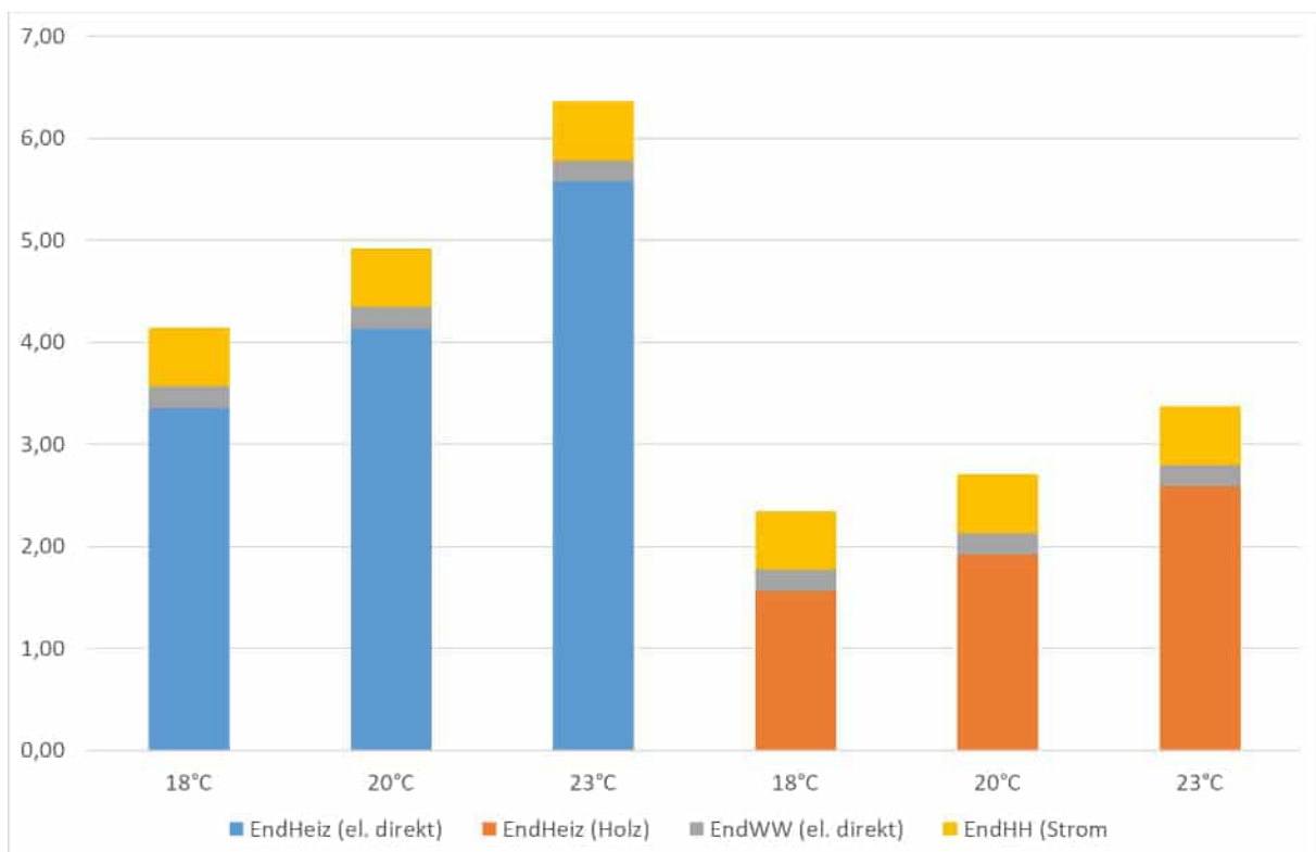
Abbildung 65: flächenspezifische, monatliche Brutto-Energiekosten des großen Gebäudes vor Sanierung gemäß Verbrauchsprognoseberechnungen PHPP unter Annahme unterschiedlicher Mittelwerte der Raumlufttemperatur in der Heizperiode für eine direkt-elektrische Beheizung aller Wohnungen und eine Beheizung aller Wohnungen über Holzöfen (in EUR/m 2 WNF pro Monat)
