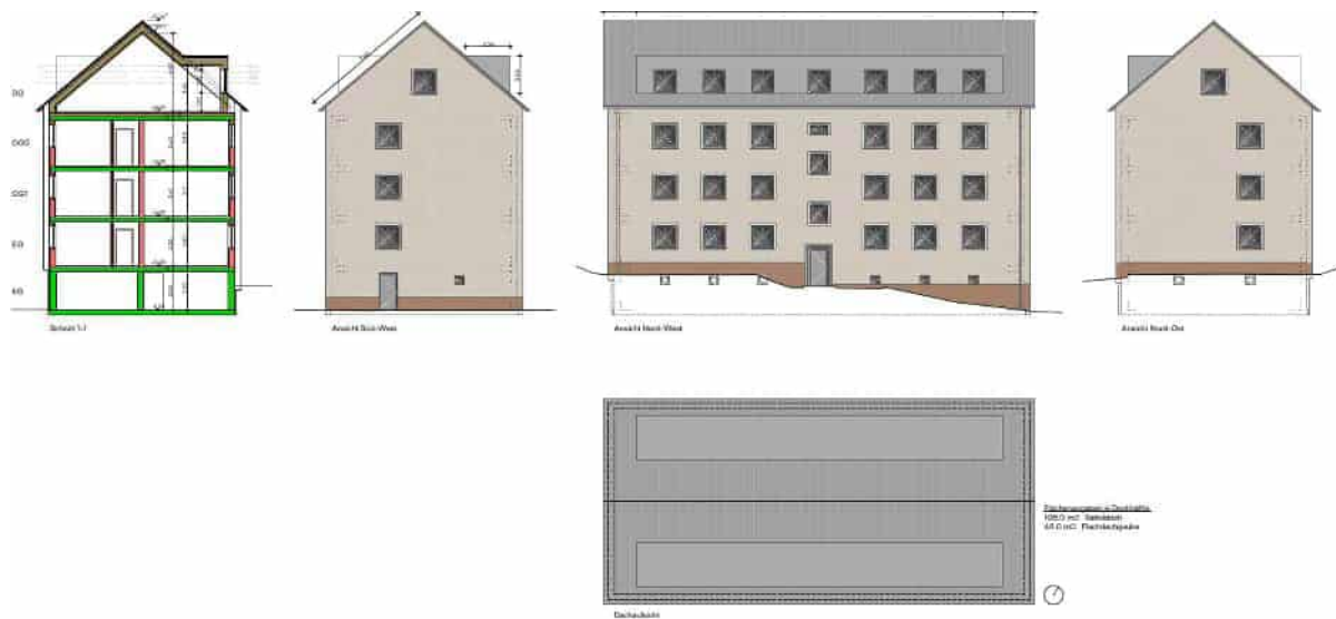
Abbildung 71: Entwurfsvarianten Dachgeschoß größeres Gebäude ohne Aufschiebling und mit großer Flachdachgaube; Johannes Kaufmann und Partner GmbH
