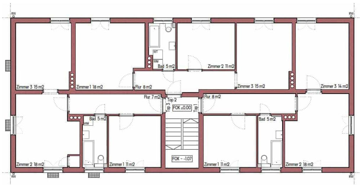
Abbildung 36: großes Gebäude, Grundriss EG, ohne Maßstab; Johannes Kaufmann und Partner GmbH
