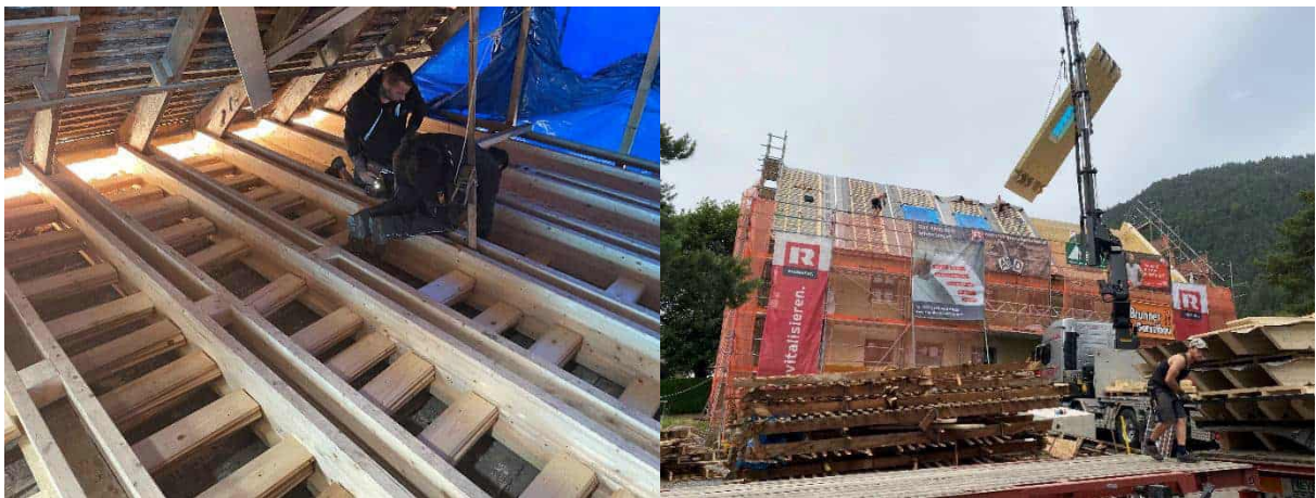
Abbildung 10: statische Verstärkung der obersten Geschoßdecke und Montage der neuen Dachelemente, kleines Gebäude; Fotos Rhomberg Bau GmbH
