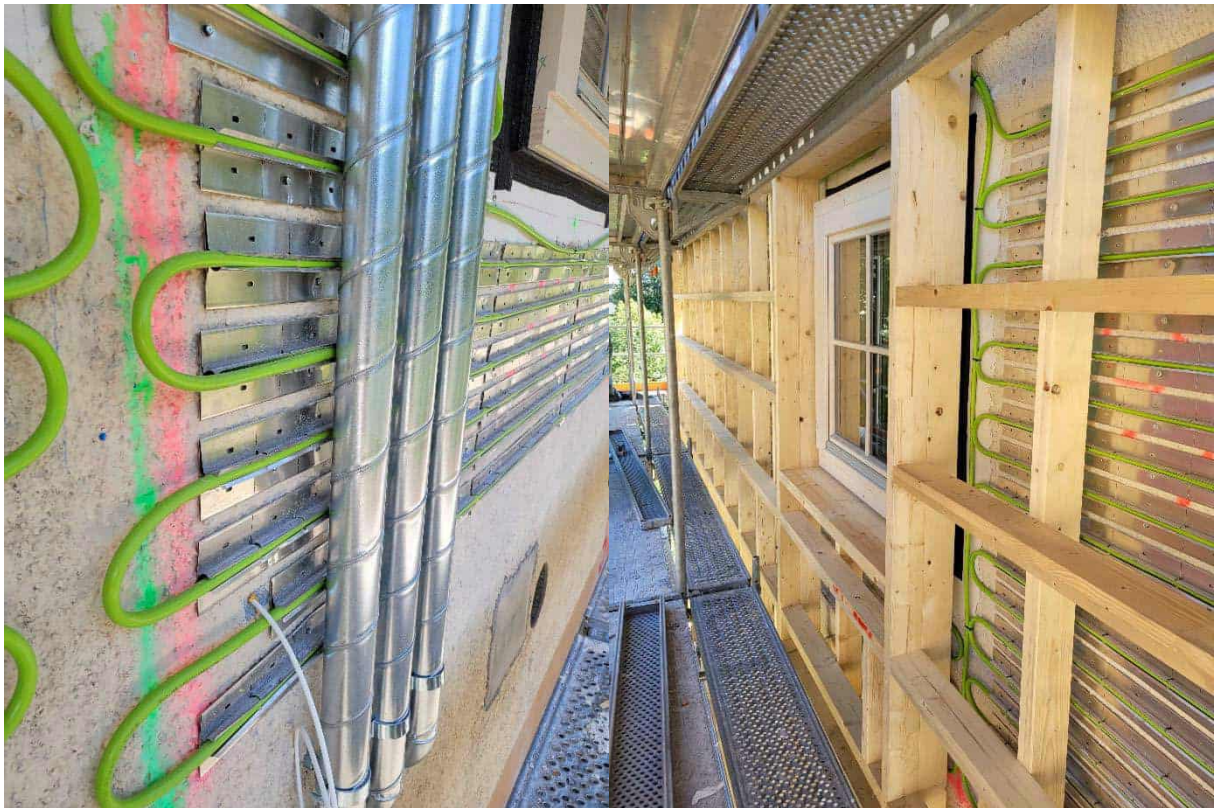
Abbildung 11: Außenwandheizung und Zuluftverteilung in Fassadenebene; teil-vorgefertigte Fassadenelemente, großes Gebäude; Fotos: Energieinstitut Vorarlberg
