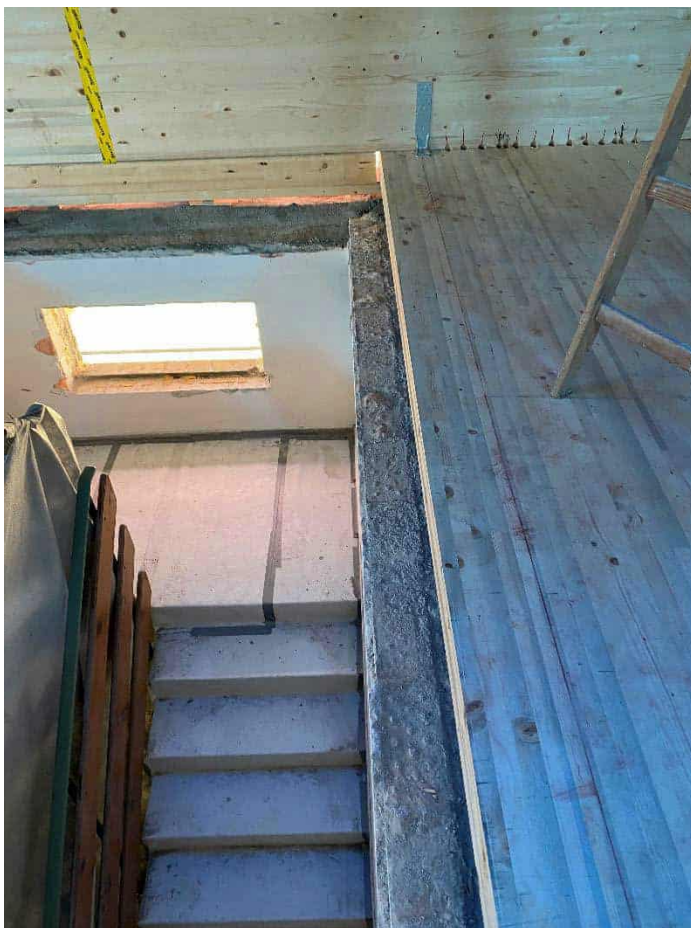
Abbildung 119: Neue lastabtragende BSH-Massivholzdecke im DG des großen Gebäudes; Foto: Rhomberg Bau GmbH
