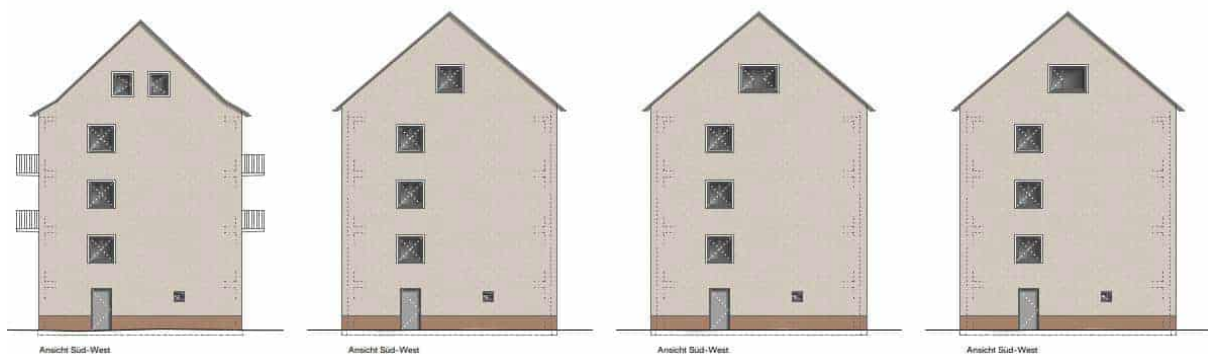
Abbildung 73: Fassadenvarianten Süd-West der Entwurfsvarianten für das Dachgeschoß des größeren Gebäudes; Johannes Kaufmann und Partner GmbH
