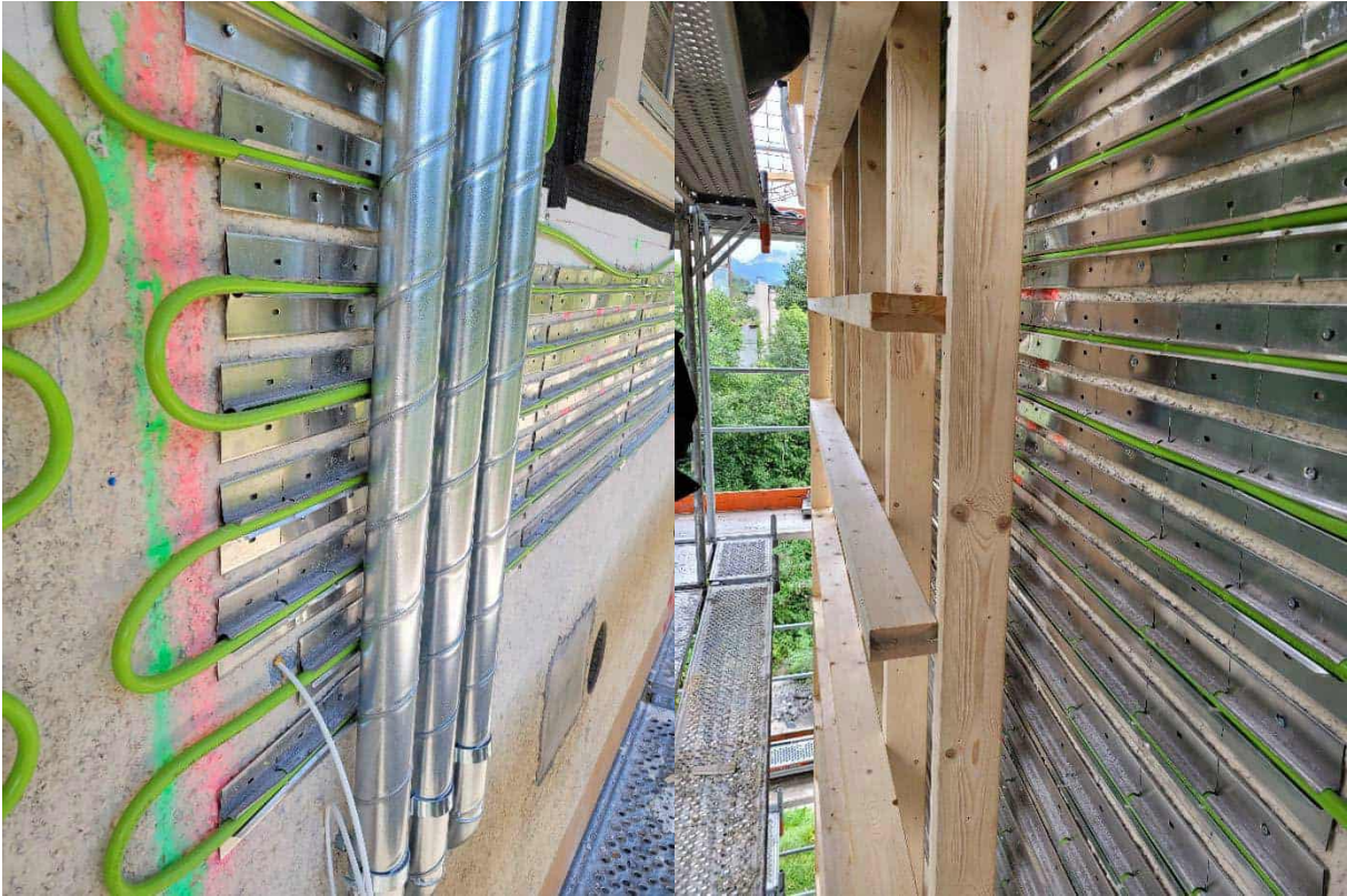
Abbildung 109: großes Gebäude: Wandheizelemente und Zuluftröhre – links; vorgefertigte Kreuzlagenelemente; Fotos: Energieinstitut Vorarlberg
