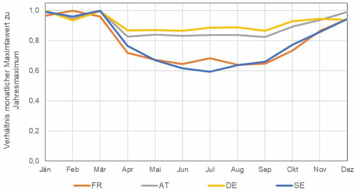
Abbildung 20: Verhältnis der maximalen Last im Mittel der Jahre 2018 und 2019 zur maximalen Last pro Monat in sechs europäischen Staaten [Büchele 2022]
