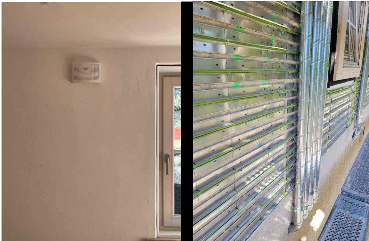
Abbildung 134: Zuluftventil an der Außenwand eines Raumes; raumweise Vertikalverteilung der Zuluft in der Ebene der Fassadenelemente; Fotos: Energieinstitut Vorarlberg
