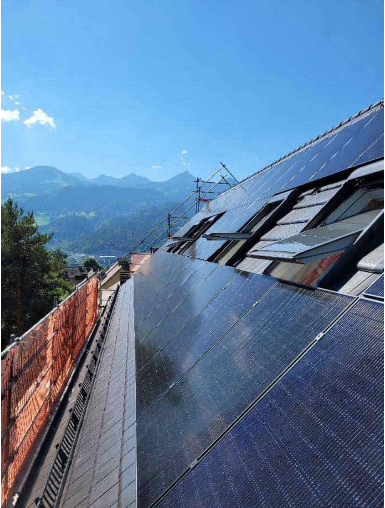
Abbildung 200: PV-Anlage kleineres Gebäude mit Dachflächenfenstern, Energieinstitut Vorarlberg
