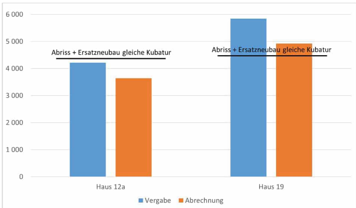
Abbildung 228: Vergleich der abgerechneten Netto-Errichtungskosten für die Sanierung der beiden Mustergebäude mit den Kosten der Option Abriss und Neubau in gleicher Kubatur und gleicher energetischer und ökologischer Qualität
